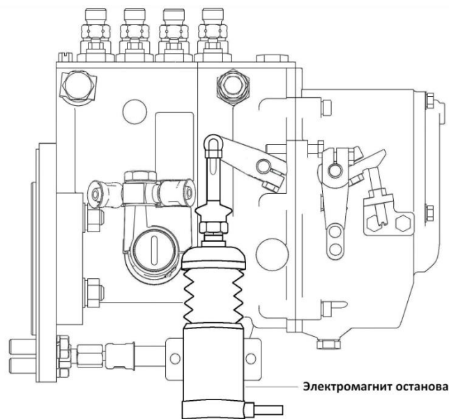
Рисунок 10 – Топливный насос высокого давления РР4М10Р1f с электромагнитом останова (фирмы «Моторпал», Чехия).
