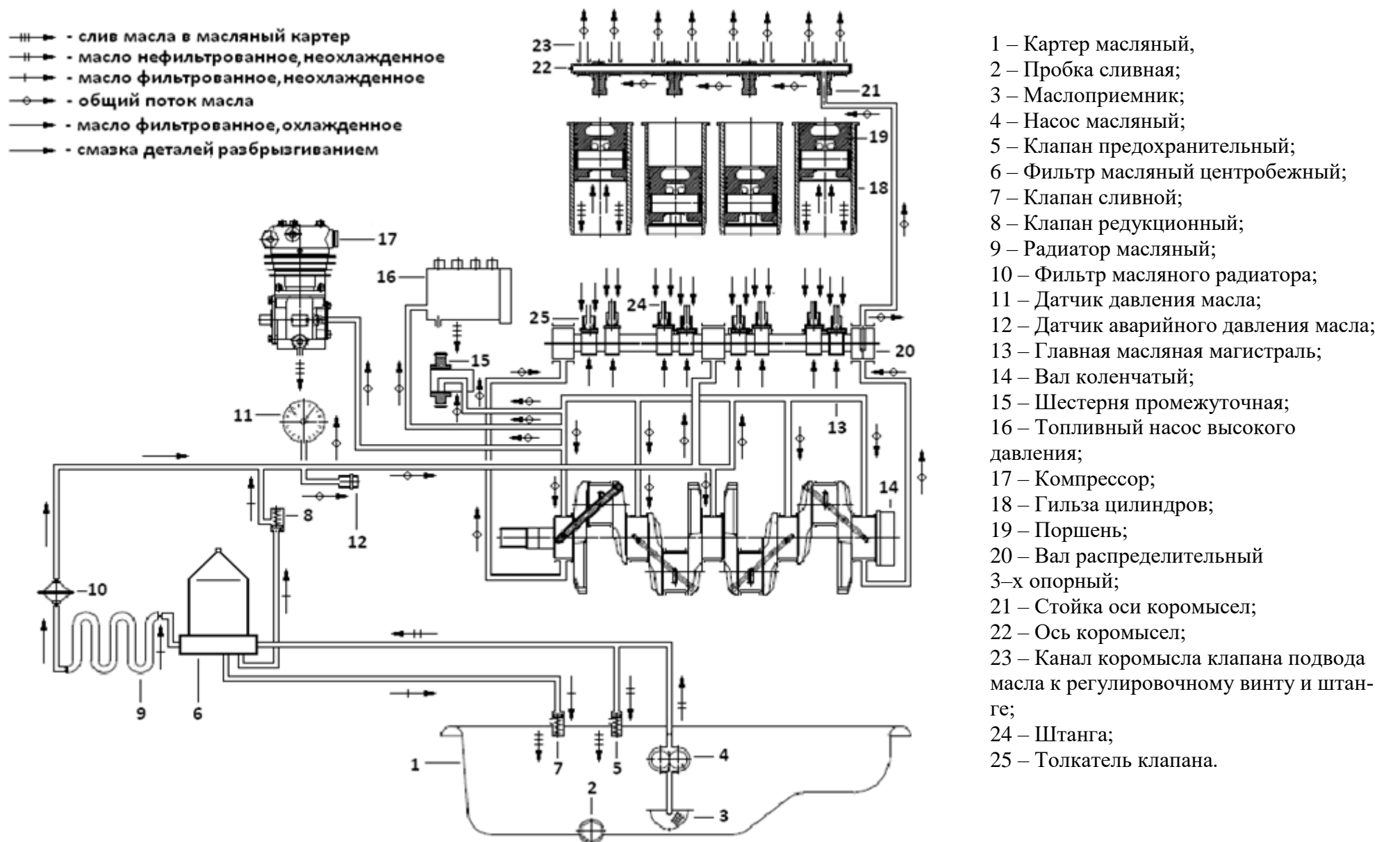
Рисунок 14 – Система смазки с центробежным масляным фильтром (ЦМФ) и масляным радиатором
