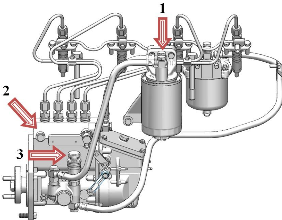
Рисунок 32 – Схема прокачки топливной системы
