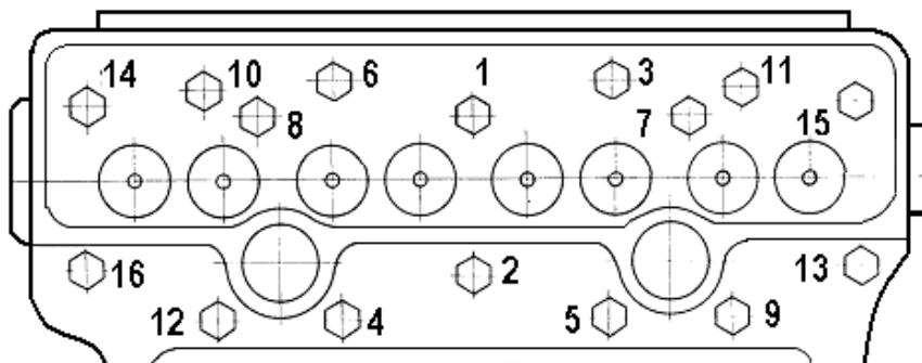
Рисунок 41 – Схема последовательности затяжки болтов крепления головки цилиндров.
