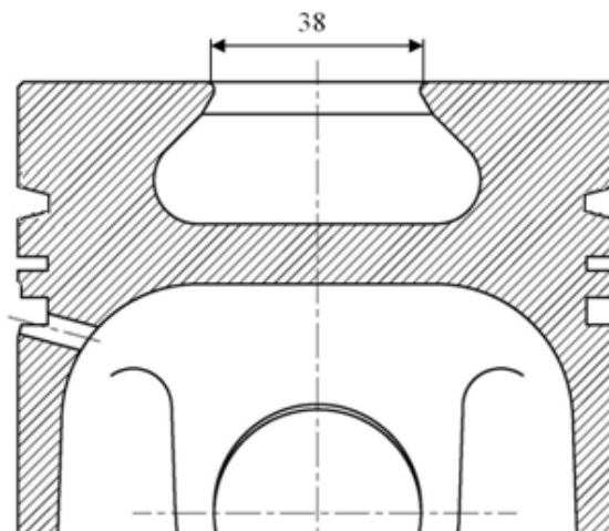
Рисунок 3 – Поршень с камерой сгорания типа Б
