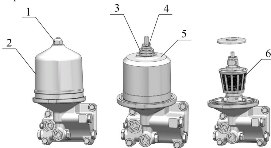
Рисунок 24 – Очистка ротора центробежного масляного фильтра
