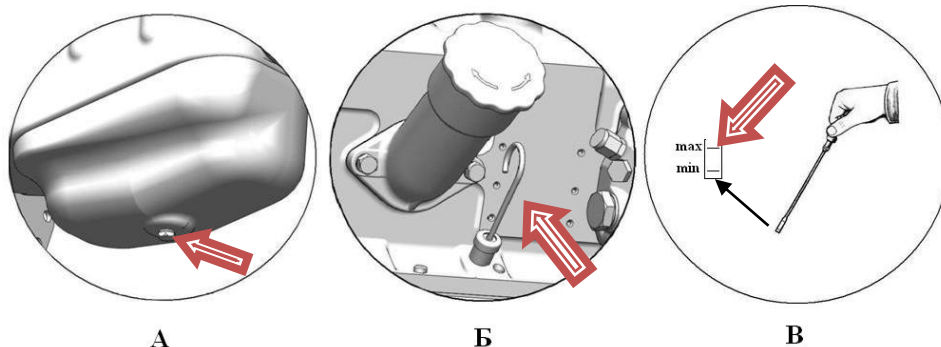
Рисунок 21 – Порядок замены масла в картере дизеля
