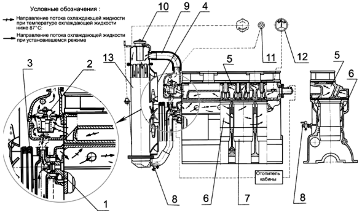
Рисунок 12 – Схема системы охлаждения дизеля (без ЖМТ).
