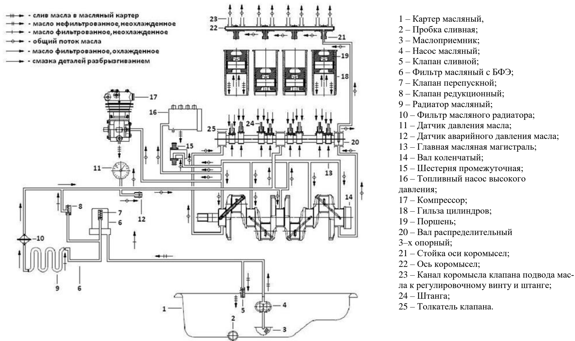
Рисунок 15 – Схема системы смазки с масляным радиатором и масляным фильтром
