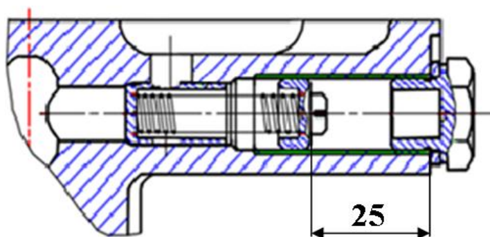
Рисунок 28 – Максимально допускаемый размер
