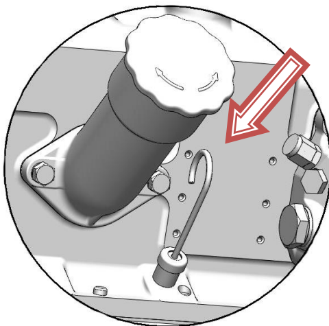
Рисунок 18 – Проверка уровня масла в картере дизеля.
