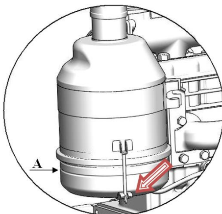
Рисунок 25 – Проверка уровня масла в поддоне воздухоочистителя
