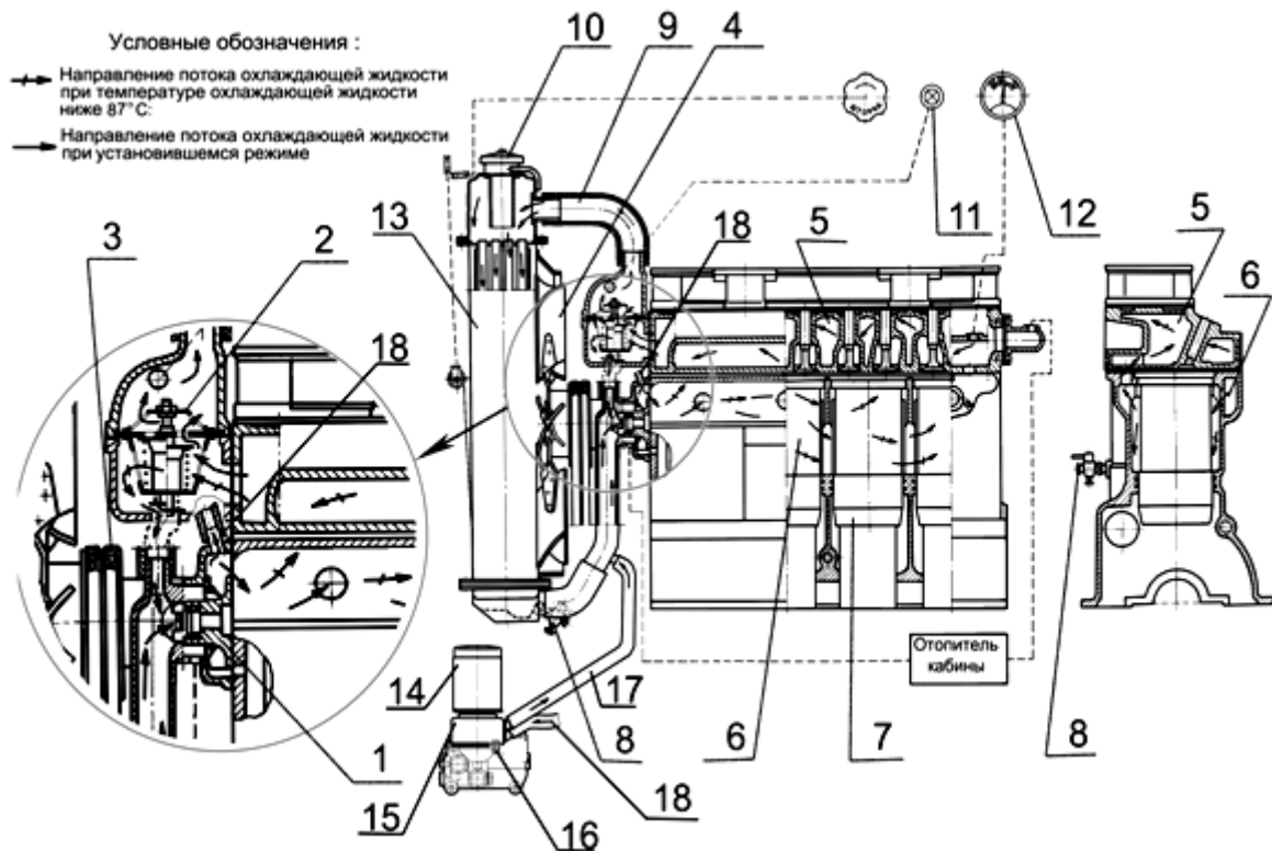
Рисунок 13 – Схема системы охлаждения дизеля с жидкостно- масляным теплообменником.
