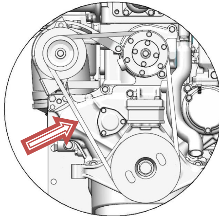
Рисунок 20 – Проверка натяжения ремня вентилятора
