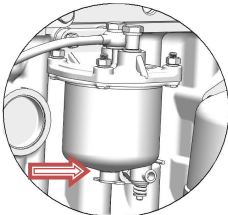
Рисунок 19 – Слив отстоя из фильтра тонкой очистки топлива
