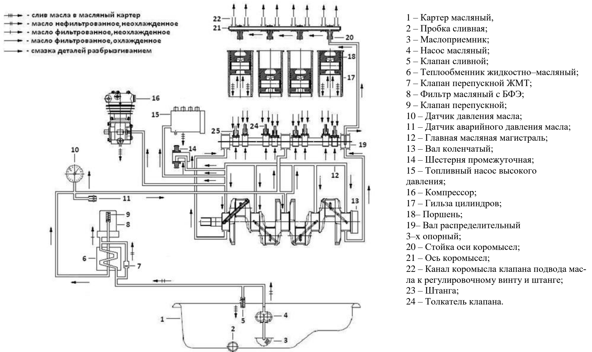
Рисунок 16 – Схема системы смазки со сменным масляным фильтром с бумажным фильтрующим элементом и жидкостно – масляным теплообменником (ЖМТ)
