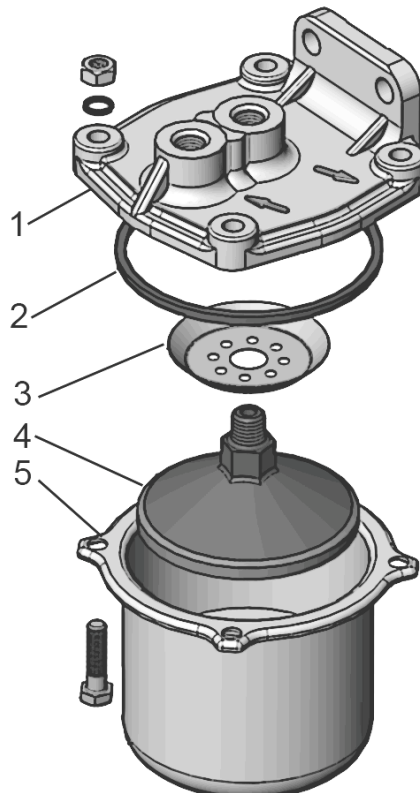
Рисунок 33 – Промывка фильтра грубой очистки топлива
