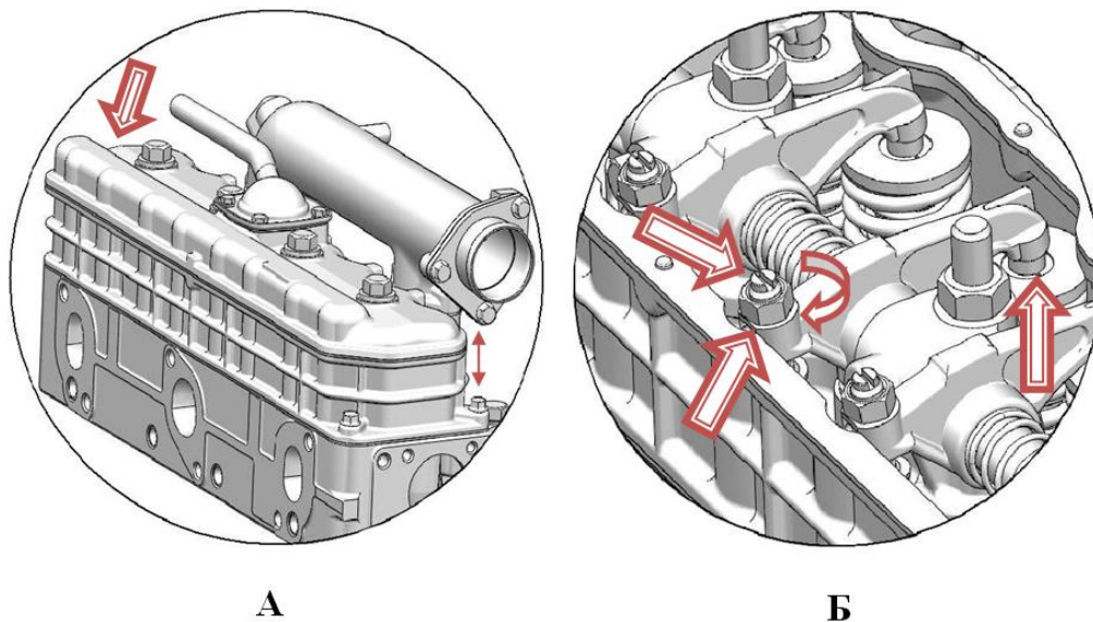
Рисунок 29 – Регулировка зазора в клапанах
