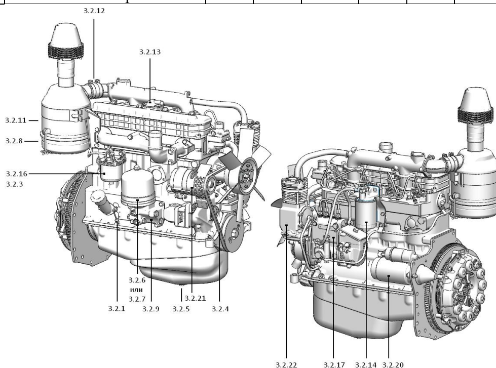
Рисунок 17 – Обслуживание составных частей дизеля
