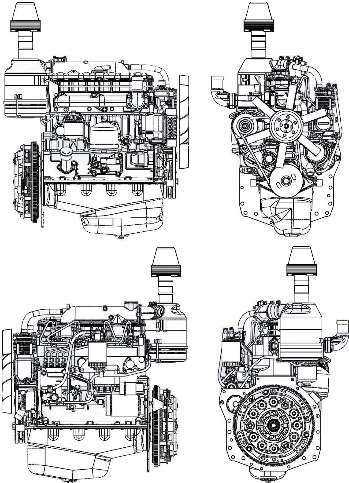
Рисунок 1 – Дизель Д-243.
